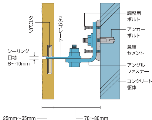
〔金物（アングルファスナー、2次式プレート）取付例〕
