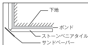
突きつけて貼り合わせ、角をサンドペーパーで軽く削る工法
