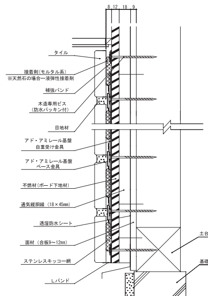
縦断面図
