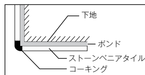
コーキングで仕上げる工法
