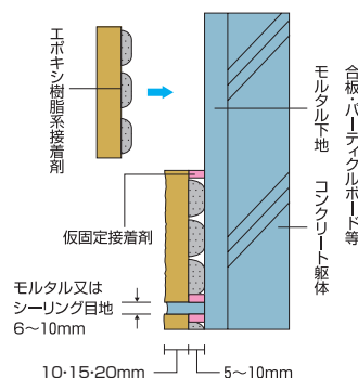
〔エポキシ系樹脂圧着貼り工法〕
