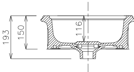
立面図
