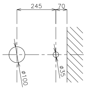
カウンター開口寸法
