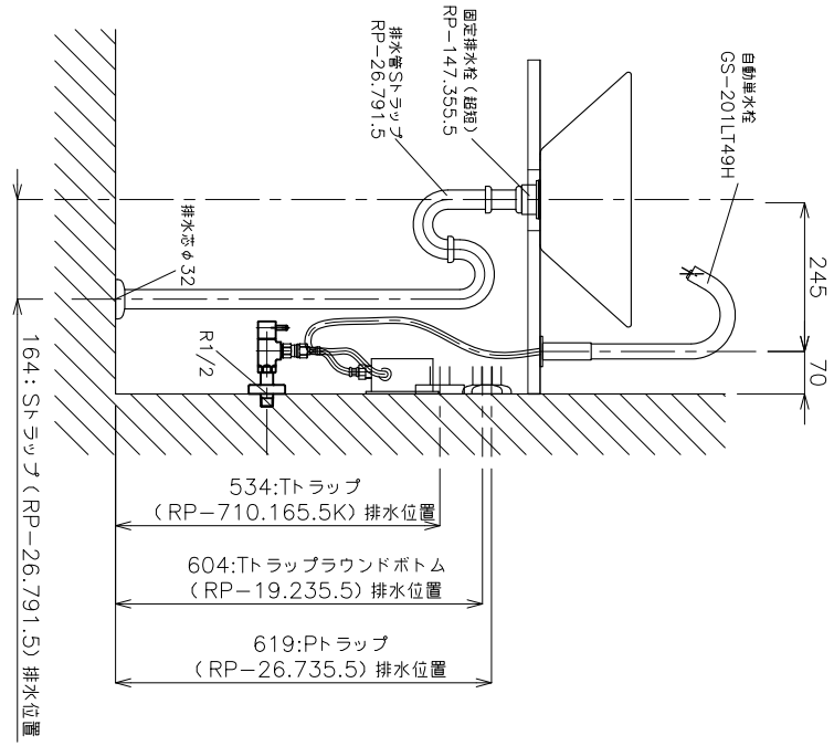
側面図
