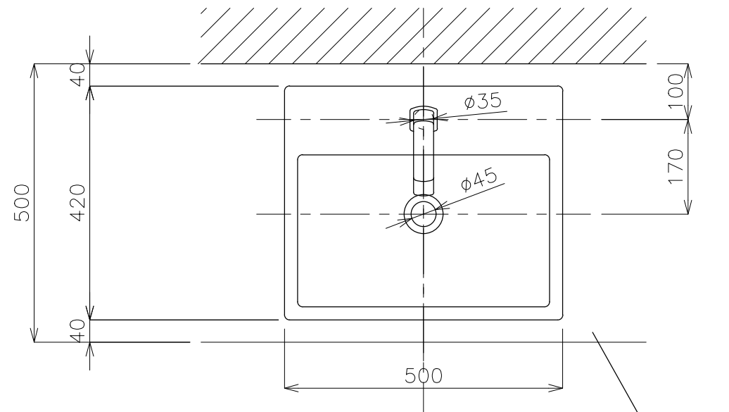
洗面ボウル GIF-607 平面図
