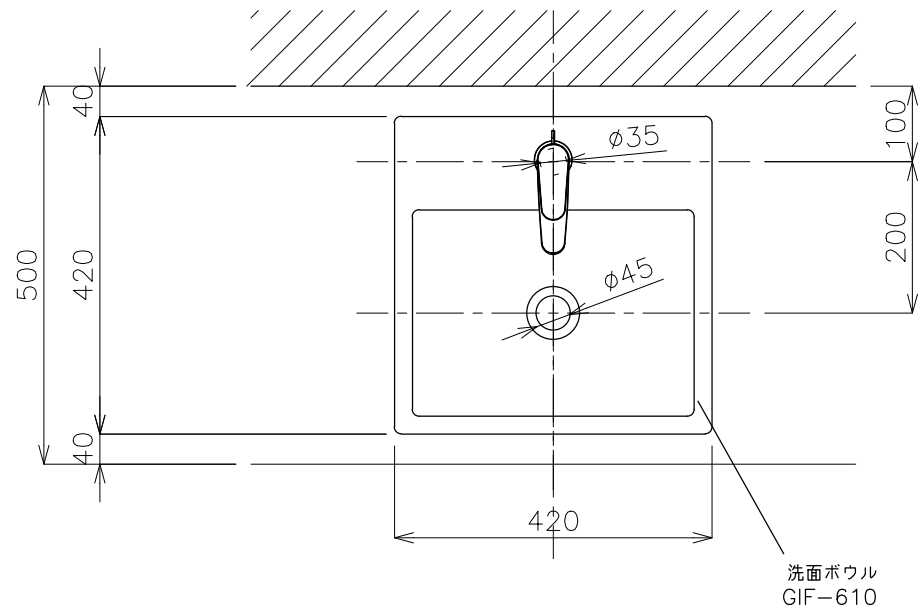
平面図
