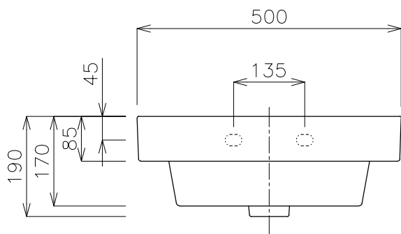
立面図
