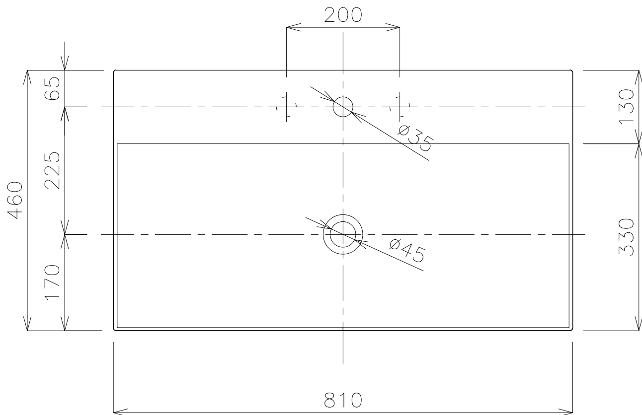
平面図
