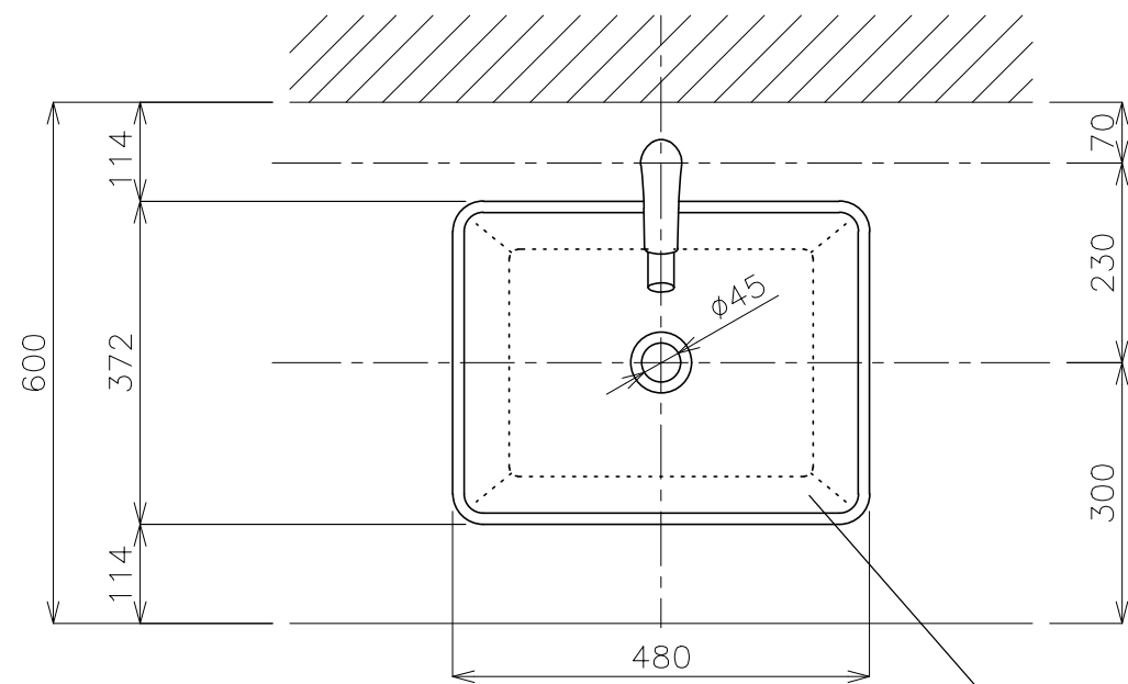
洗面ボウル GIF-852 平面図
