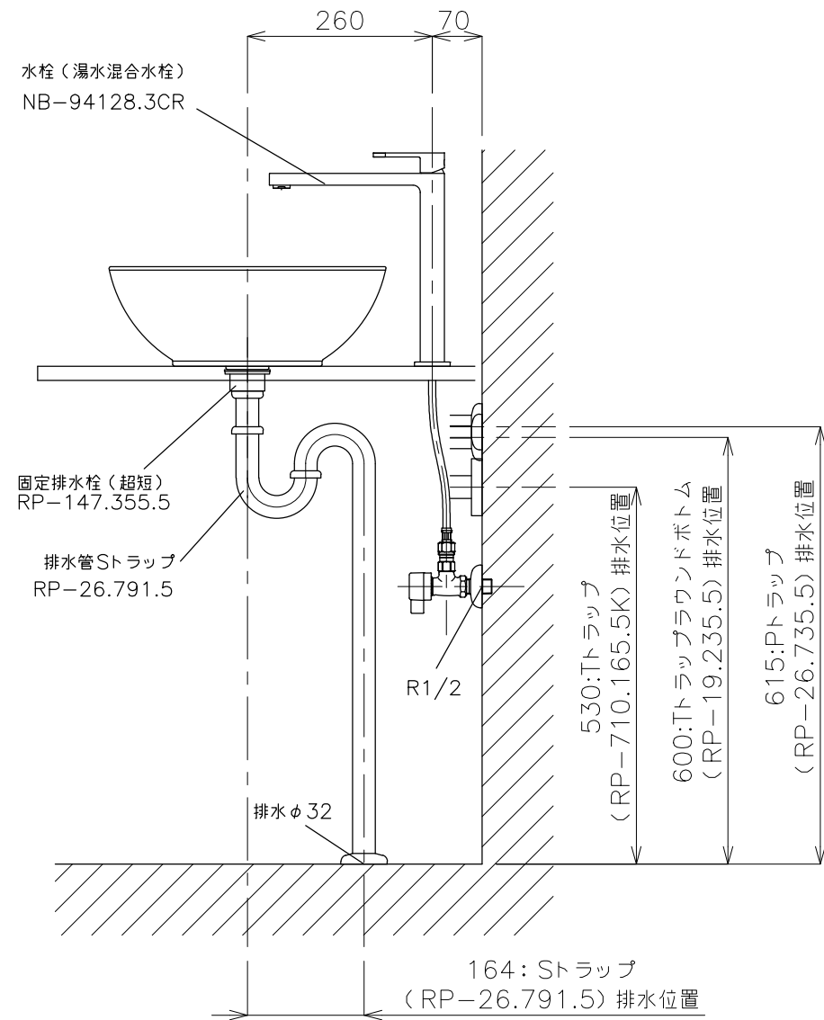
側面図
